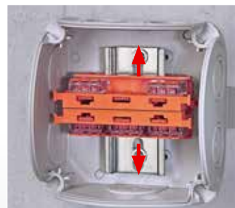
Forskellige klemmepositioner på præmonteret DIN-skinne
